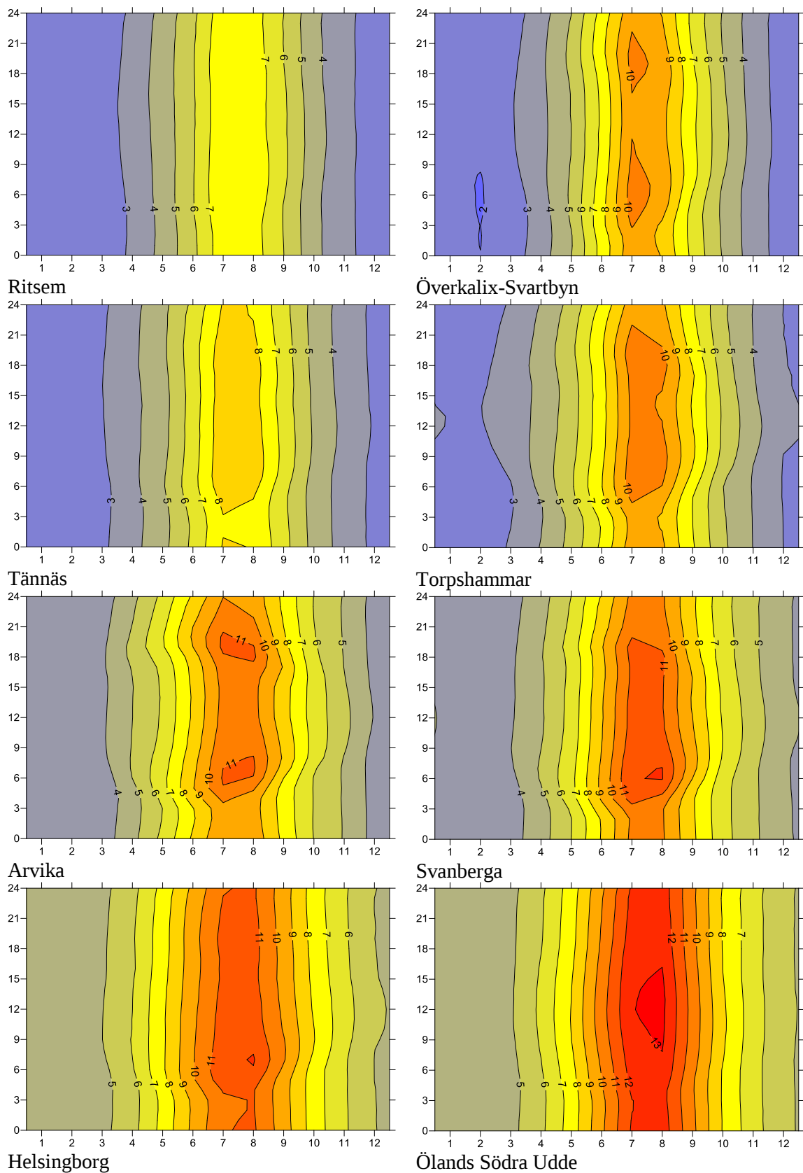
Figur 44. Absolut fuktighet [ g\text{ vatten}/m^3 ], variation under månad (x-axel) och under dygn (y-axel), medelvärden 1996-2012.
