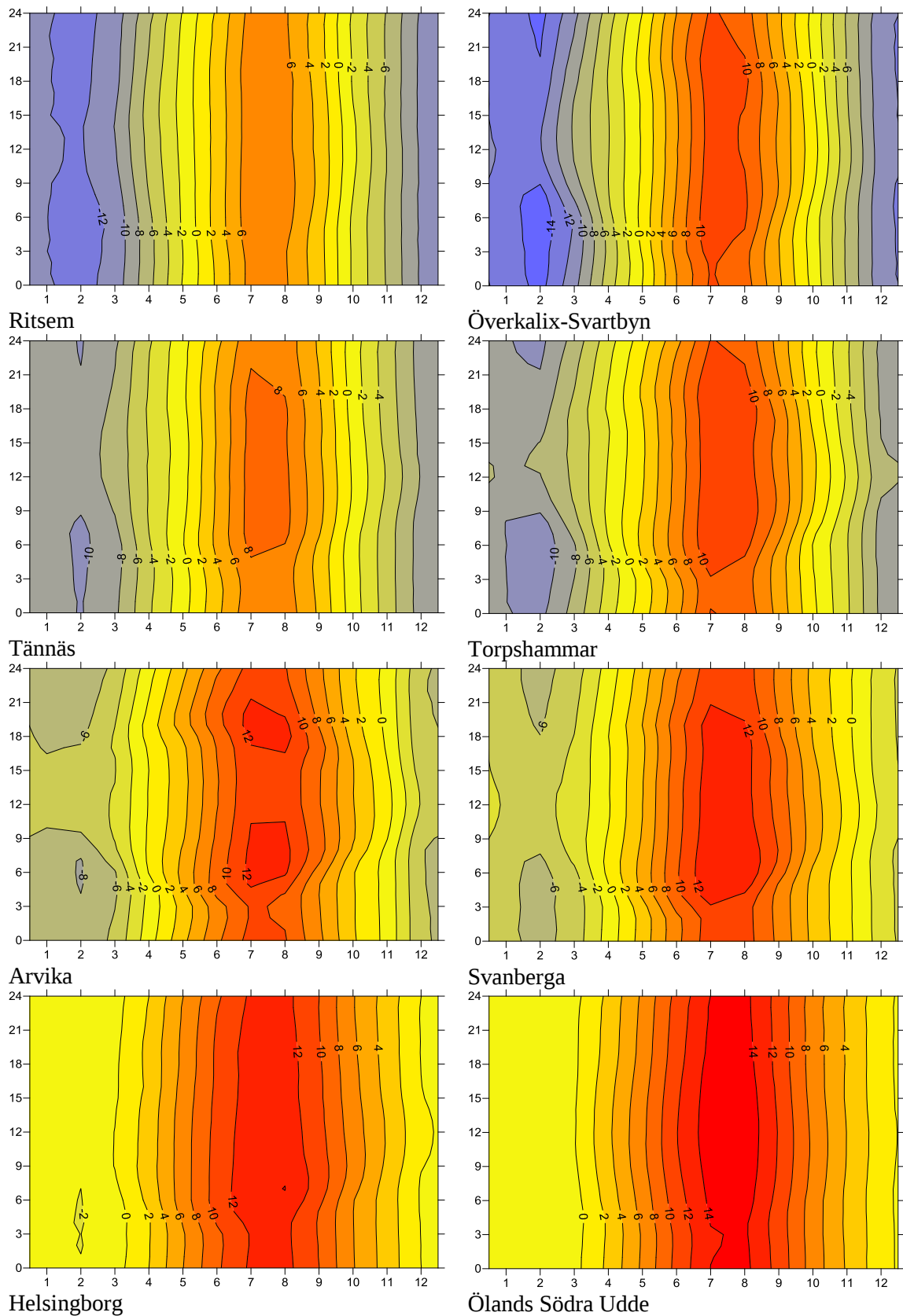
Figur 41. Daggpunkt [ ^{\circ}\text{C} ], variation under månad (x-axel) och under dygn (y-axel), medelvärden 1996-2012.
