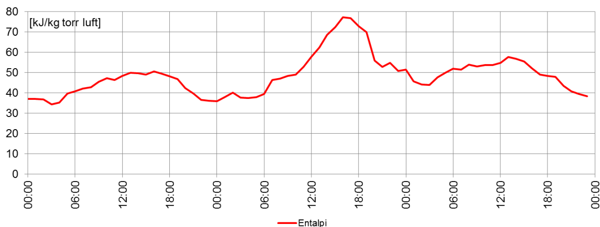
Figur 20. Enthalpi. Hällum 1997-06-29 - 1997-07-01.
