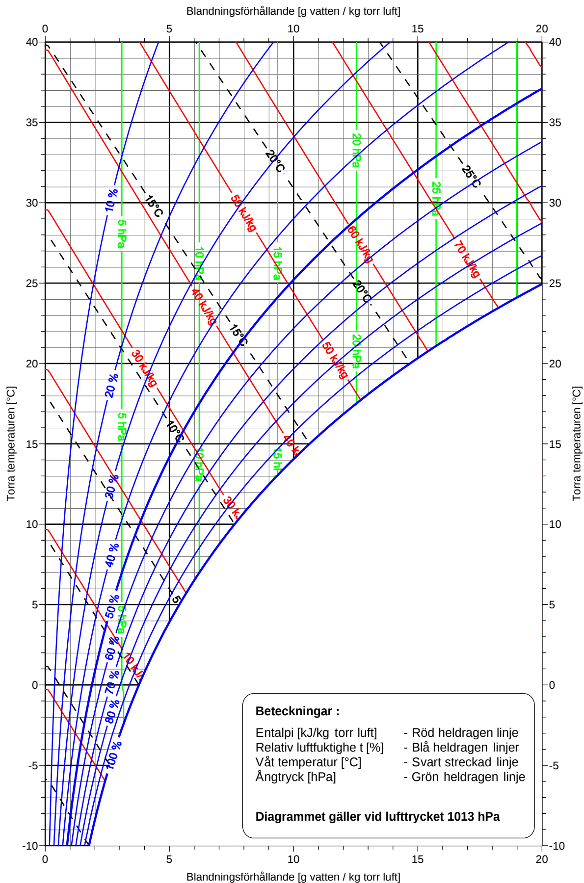
Figur 25. Mollierdiagram för fuktig luft.
