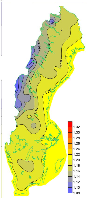
Figur 38. Luftens densitet [ \text{kg/m}^3 ], medelvärden 1996-2012.
