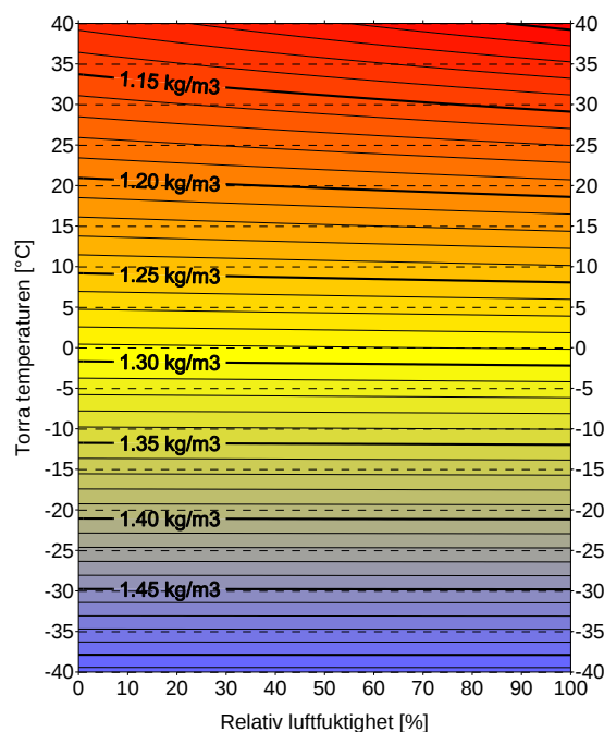
Figur 21. Hur luftens densitet beror av temperatur och relativ luftfuktighet vid lufttrycket 1013\text{ hPa} .
