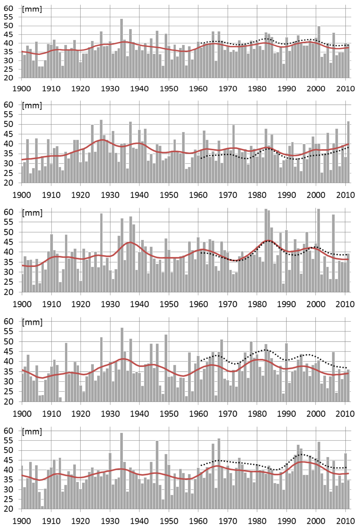
Figur 60. Höstmånadernas (september – november) medelvärde av årets största 4-dygnsnederbörd. Uppifrån och ner: Hela landet, Norra Norrland, Södra Norrland, Svealand och Götaland.
