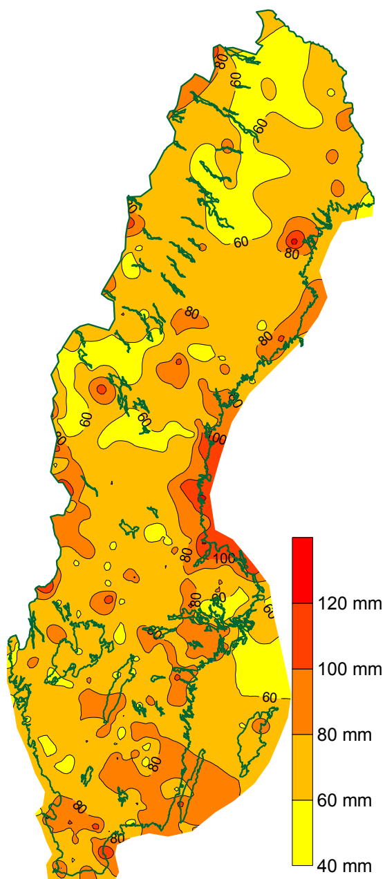
Figur 38. 100 års återkomsttid av 1-dygnsnederbörd [mm].
