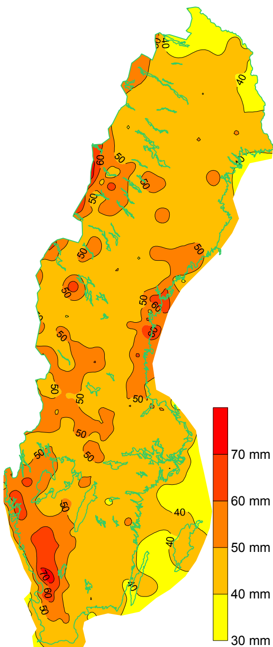
Figur 72. 1 års återkomsttid av 4-dygnsnederbörd [mm].
