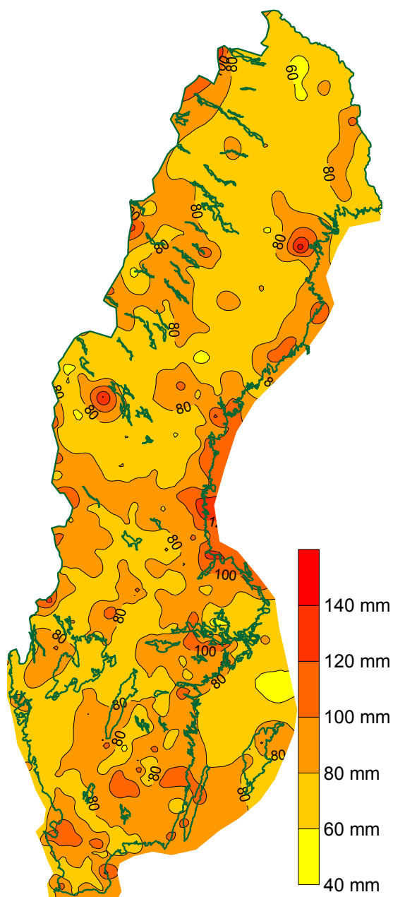
Figur 135. 100 års återkomsttid av maximal 24-timmarsnederbörd [mm].
