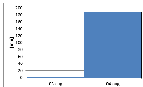
Figur 51. Dygnsnederbörd under två dygn i RÅDA.
