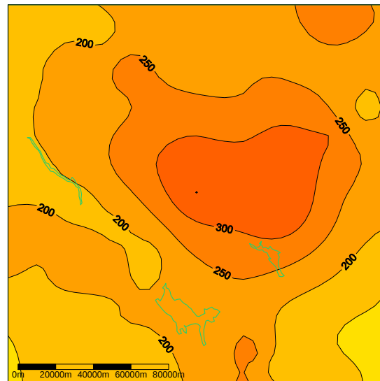
Figur 124. Nederbördssumma [mm] 2000-06-25 – 2000-07-24.
