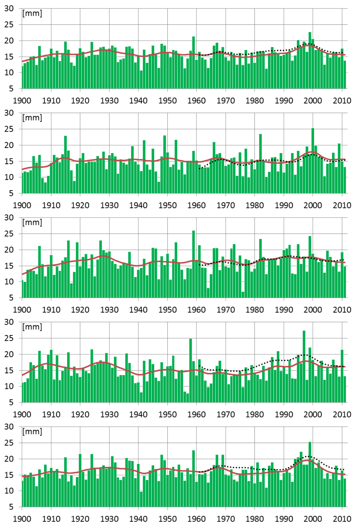
Figur 25. Varmånadernas (mars – maj) medelvärde av årets största 1-dygnsnederbörd. Uppifrån och ner: Hela landet, Norra Norrland, Södra Norrland, Svealand och Götaland.
