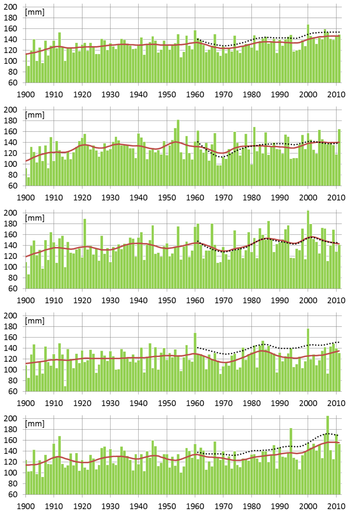
Figur 114. Medelvärdet av årets största 30-dygnsnederbörd. Uppifrån och ner: Hela landet, Norra Norrland, Södra Norrland, Svealand och Götaland.
