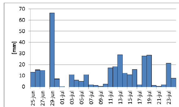
Figur 125. Dygnsnederbörd under 30 dygn i KVARNBERG.
