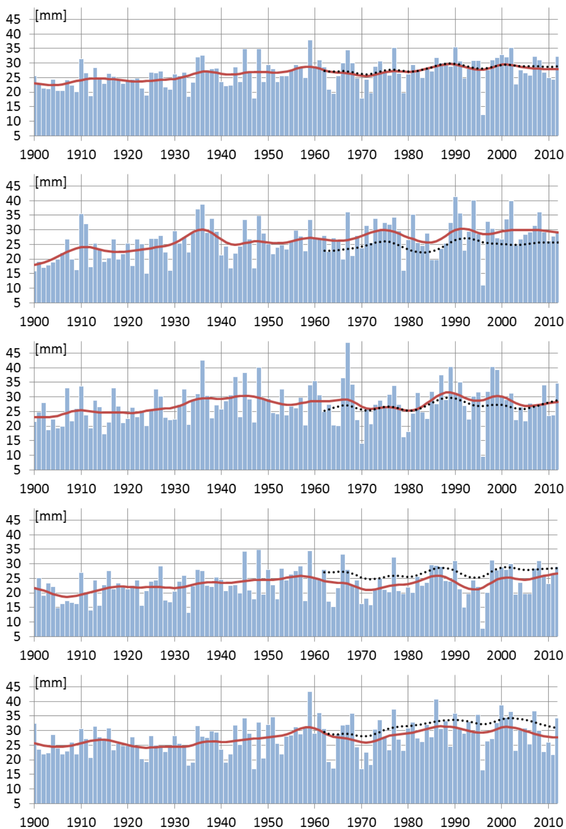
Figur 61. Vintermånadernas (december – februari) medelvärde av årets största 4-dygnsnederbörd. Uppifrån och ner: Hela landet, Norra Norrland, Södra Norrland, Svealand och Götaland.
