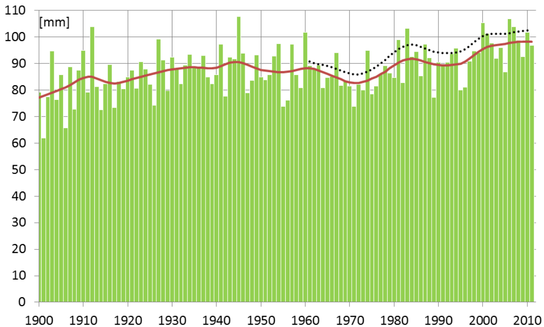
Figur 18. Medelvärde av årets största 14-dygnsnederbörd (staplar) som bygger 60 utvalda stationer. Röd kurva visar en utjämnad kurva av staplarna. Prickad svart kurva visar en utjämnad kurva baserad på nederbördsdata från samtliga stationer som varit i drift under året.
