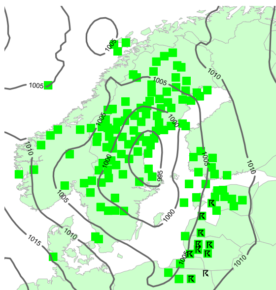
Figur 30. Väderläget 2001-08-27 kl.18 UTC. Grönt – nederbörd, gult - dimma, linjer – isobarer, ⚡ – åska
