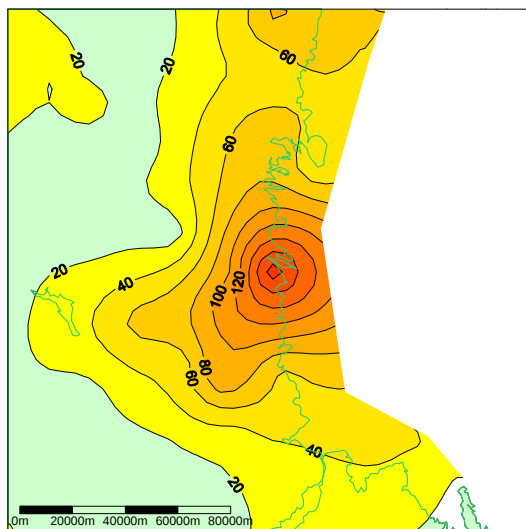
Figur 48. Nederbördssumma[mm] 1992-10-15 – 1992-10-16.
