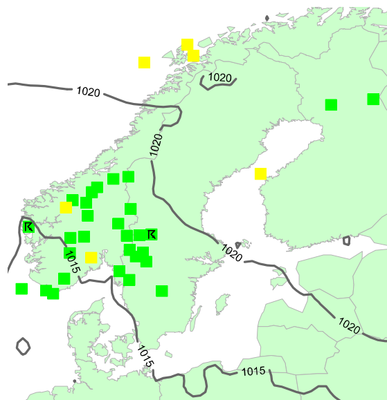
Figur 32. Väderläget 2004-08-04 kl. 18 UTC. Grönt – nederbörd, gult - dimma, linjer – isobarer, ⚡ – åska
