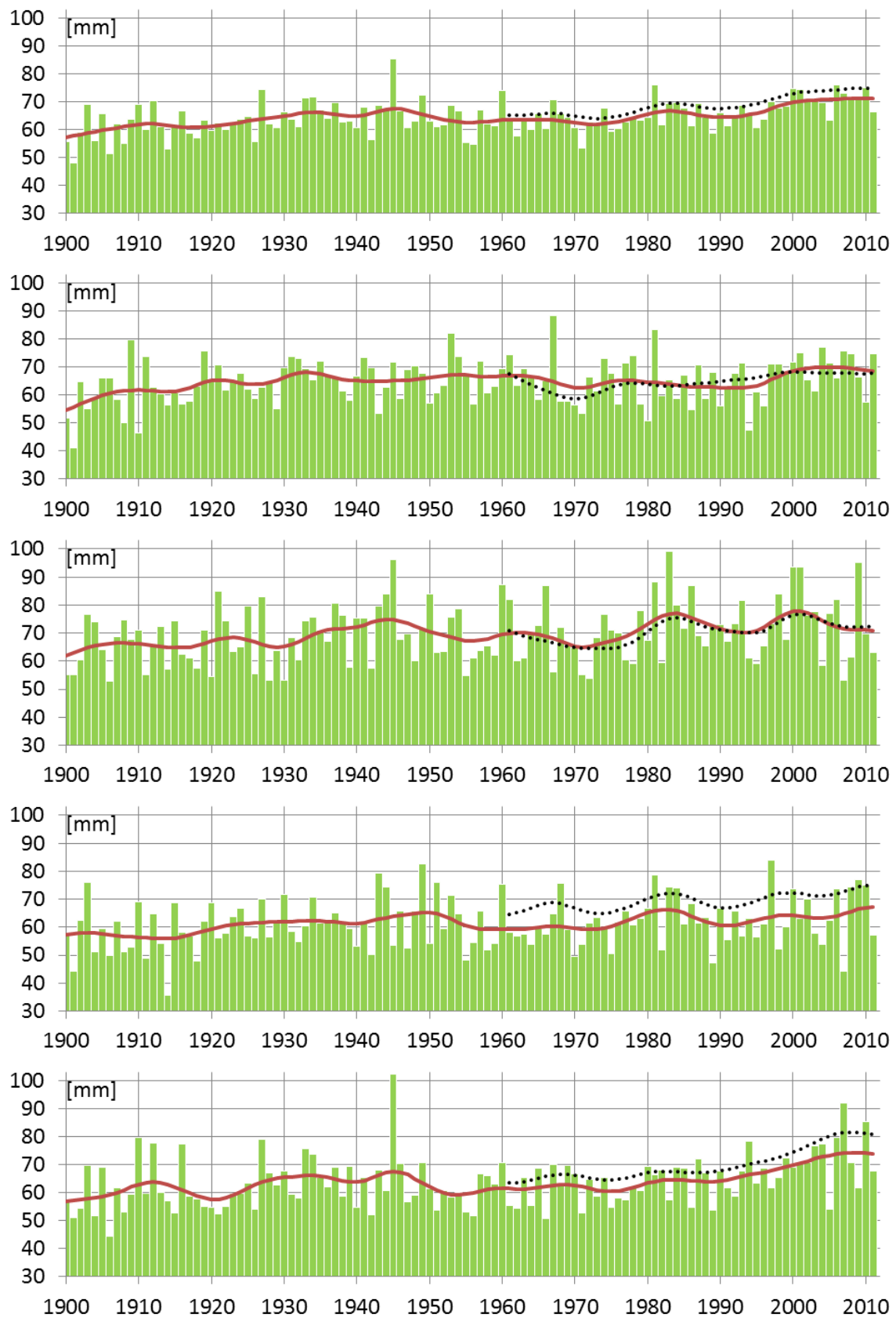
Figur 76. Medelvärdet av årets största 7-dygnsnederbörd. Uppifrån och ner: Hela landet, Norra Norrland, Södra Norrland, Svealand och Götaland.
