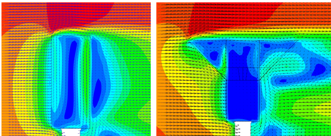
Figur 4. Strömningsberäkning kring nederbördsräkare utan vindskydd till vänster och med vindskydd till höger. Färgerna visar vindhastighet. Röd färg innebär relativt högre vindhastighet medan blå färg innebär relativt lägre.
