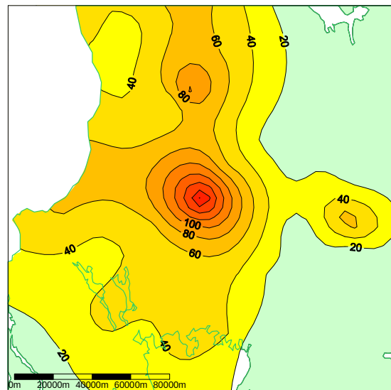
Figur 31. Nederbördssumma[mm] 2004-08-04.
