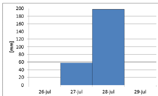
Figur 65. Dygnsnederbörd under fyra dygn i FAGERHEDEN.
