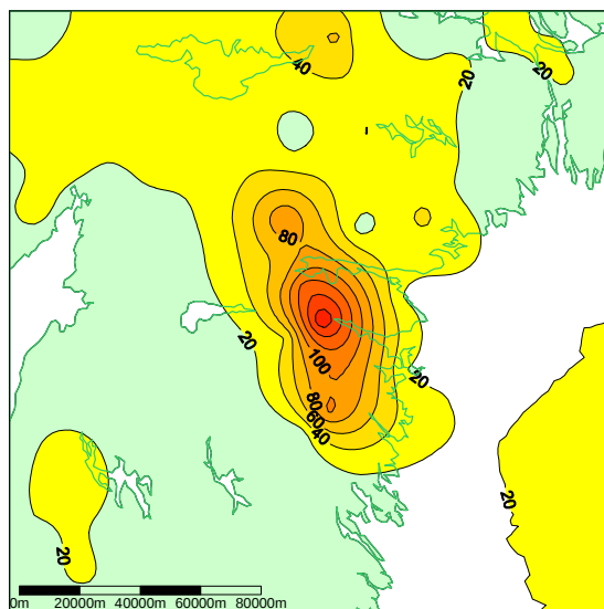
Figur 33. Nederbördssumma [mm] 1973-07-09.
