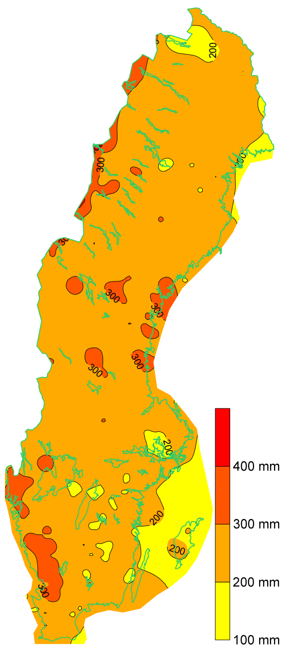
Figur 131. 100 års återkomsttid av 30-dygnsnederbörd [mm].
