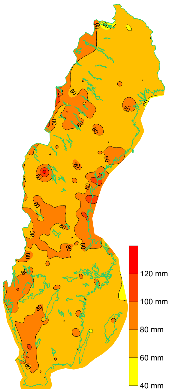
Figur 73. 10 års återkomsttid av 4-dygnsnederbörd [mm].
