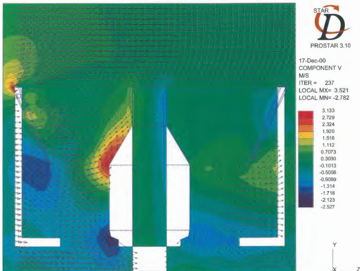
Figur A3 Strömning runt en GEONOR-kanna med Alter-vindskärm. Vindvektorn i bildplanet ges med vindpilar medan den vertikala komponenten (V i denna bild) framgår mer i detalj av färgfältet.
