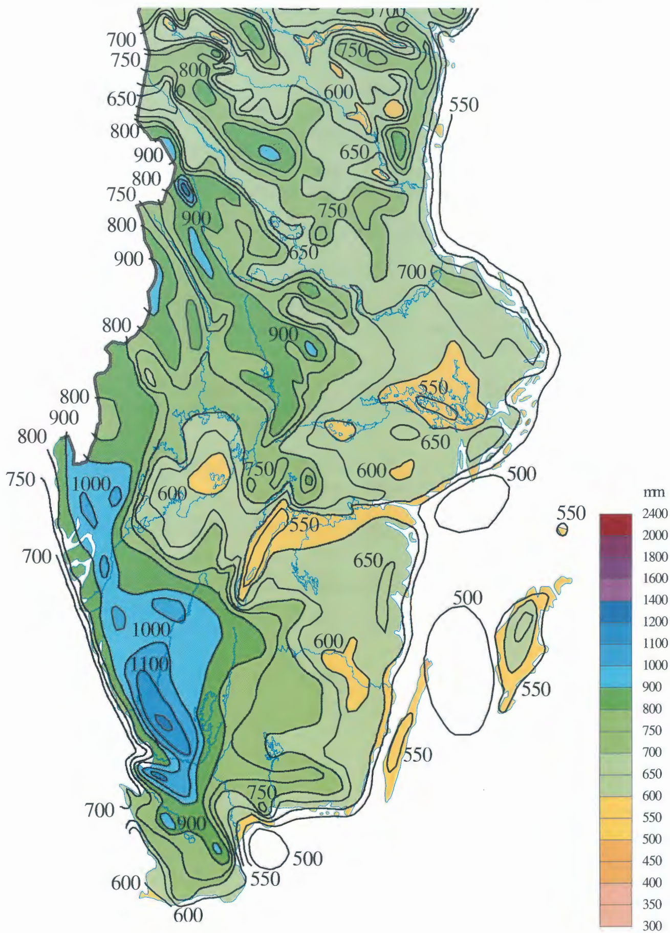
Figur 2 Korrigerad årsmedelnederbörd 1961-1990 enligt föreliggande rapport (jämför appendix 3)
