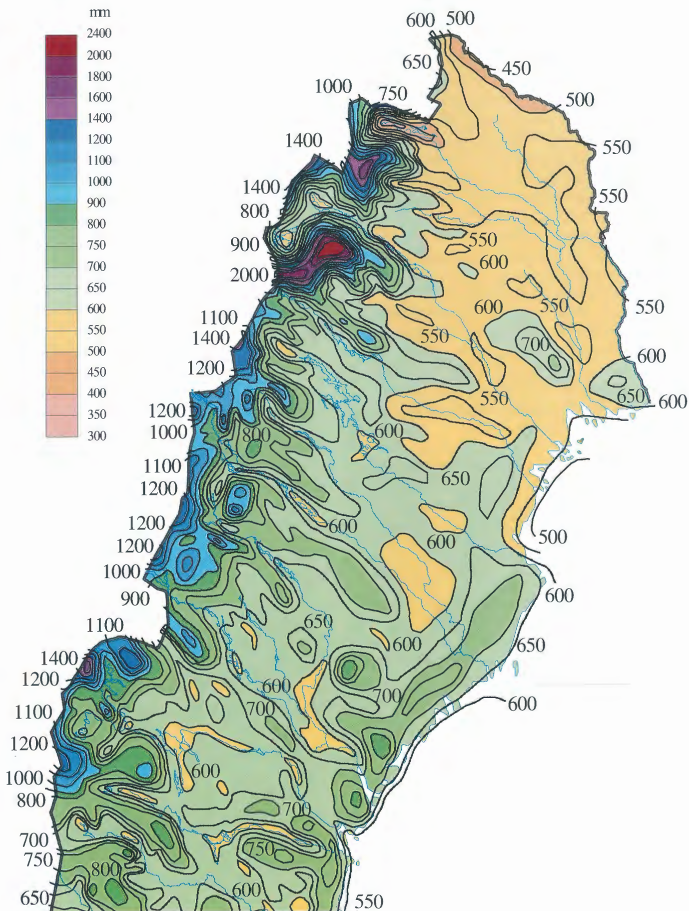
Figur 2 Korrigerad årsmedelnederbörd 1961-1990 enligt föreliggande rapport (jämför appendix 3)
